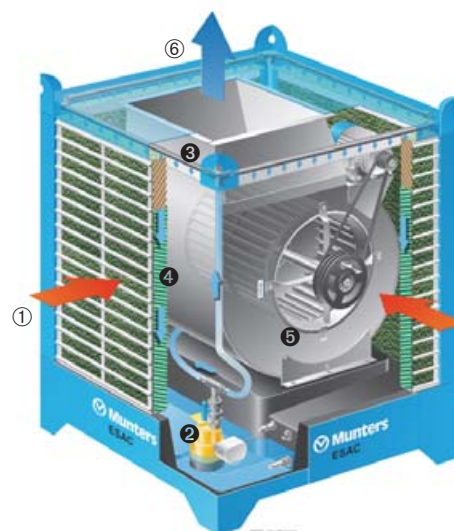
Принцип испарительного охлаждения
